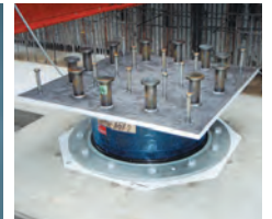
免震装置
